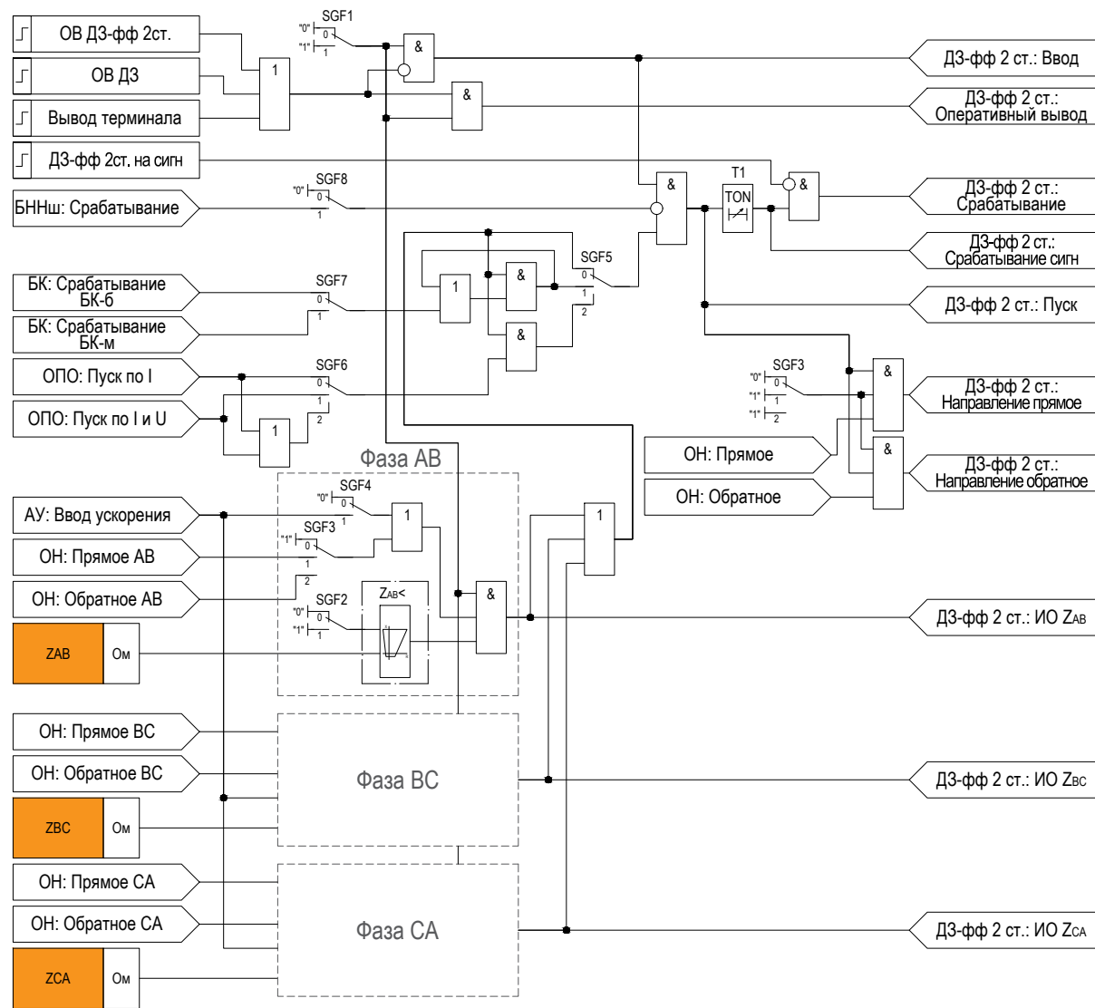
Рисунок 2.4 – Функциональная схема «Д3-фф 2ст.»
